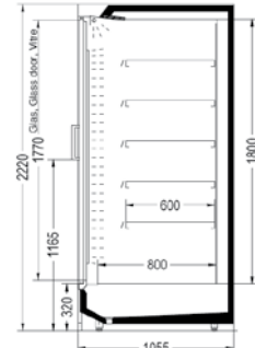
MenEco LU.HP-A L
