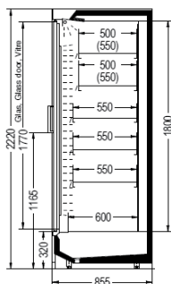
MenEco EU.HP-A L
